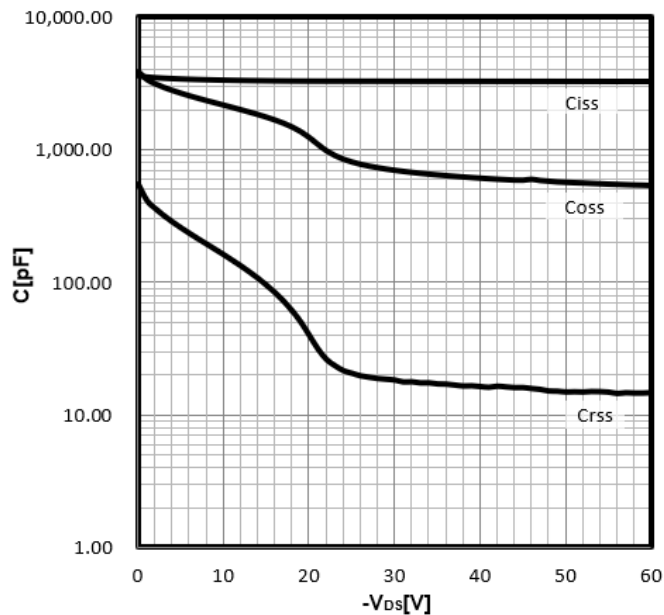
Typ. capacitances
